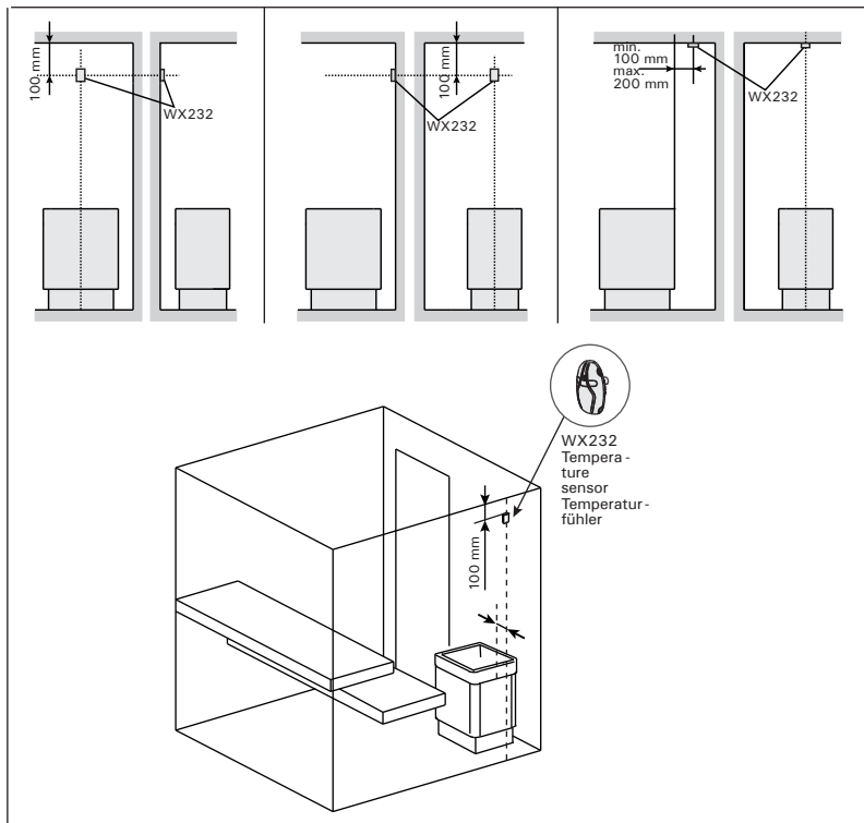
Position der Temperaturfühler bei Freistehende Öfen
