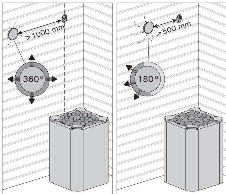
Position der Temperaturfühler bei Öfen mit Wandbefestigung
