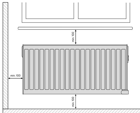
Minimivstånd vid installation
