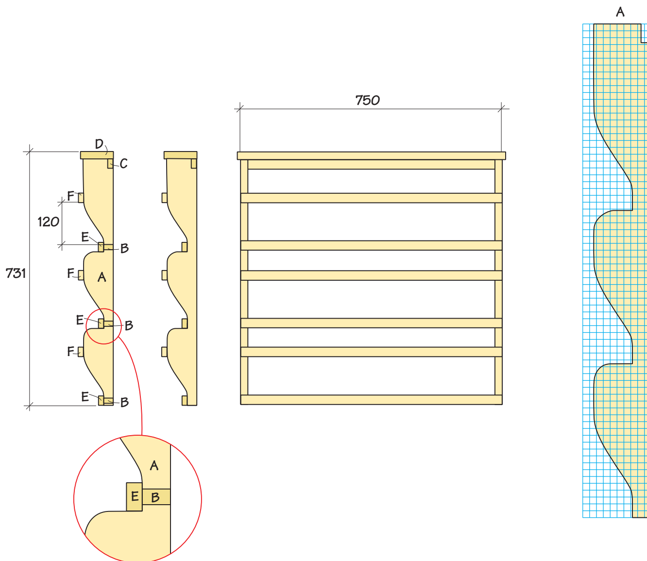
Ritning tallrikshylla
